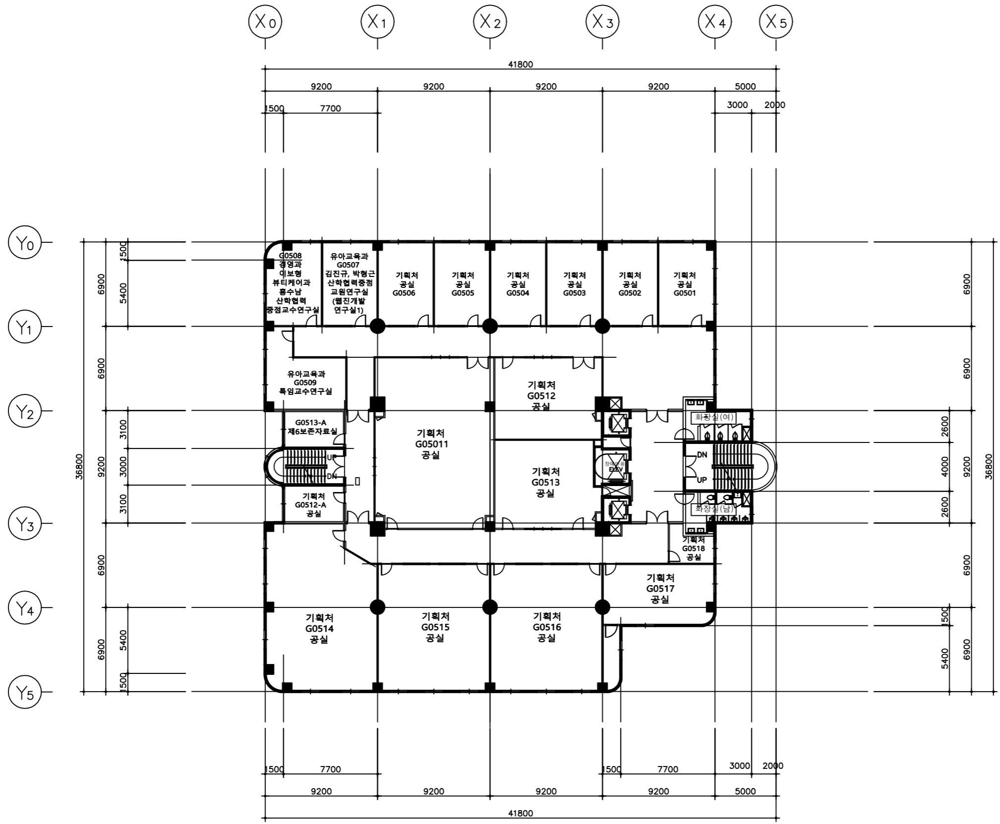
몽당도서관 5층(변경전) SCALE : 1/300
